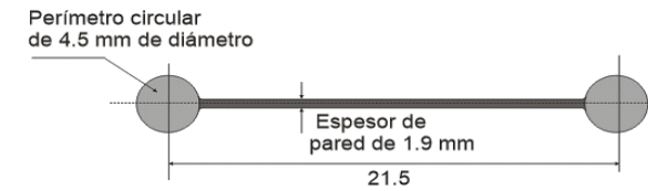
Detalle a-a:
